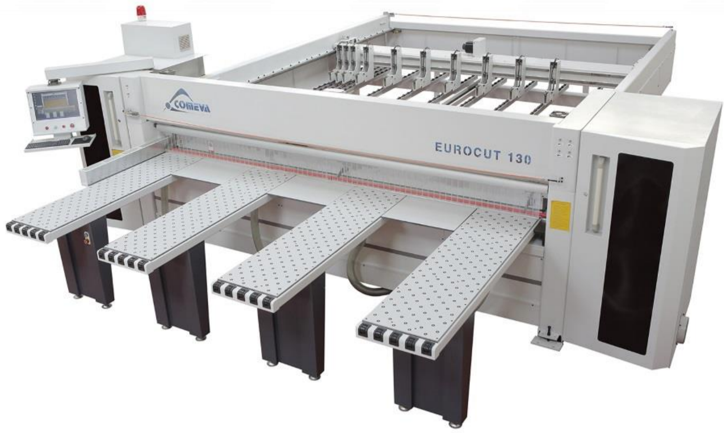
Seccionadora Automática Eurocut 130/3300
